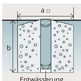
Entwässerung
